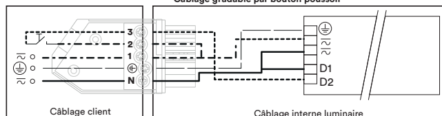
Câblage client Câblage interne luminaire
