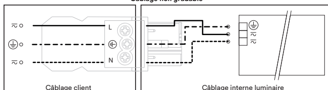
Câblage client Câblage interne luminaire
