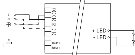
Câblage gradable par bouton poussoir pour OPERA
