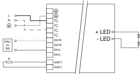
Câblage gradable par bus DALI ou DSI pour OPERA
