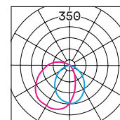
diffuseur semi- opale + réflecteur asym. ext. C0D1R2
